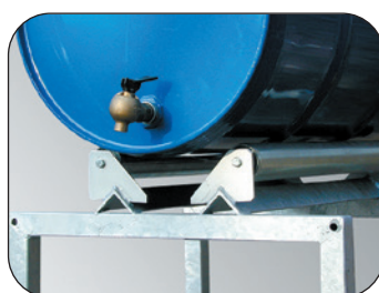
Drehbare Rollenauflage, Artikel-Nr. Z50-1925-B
